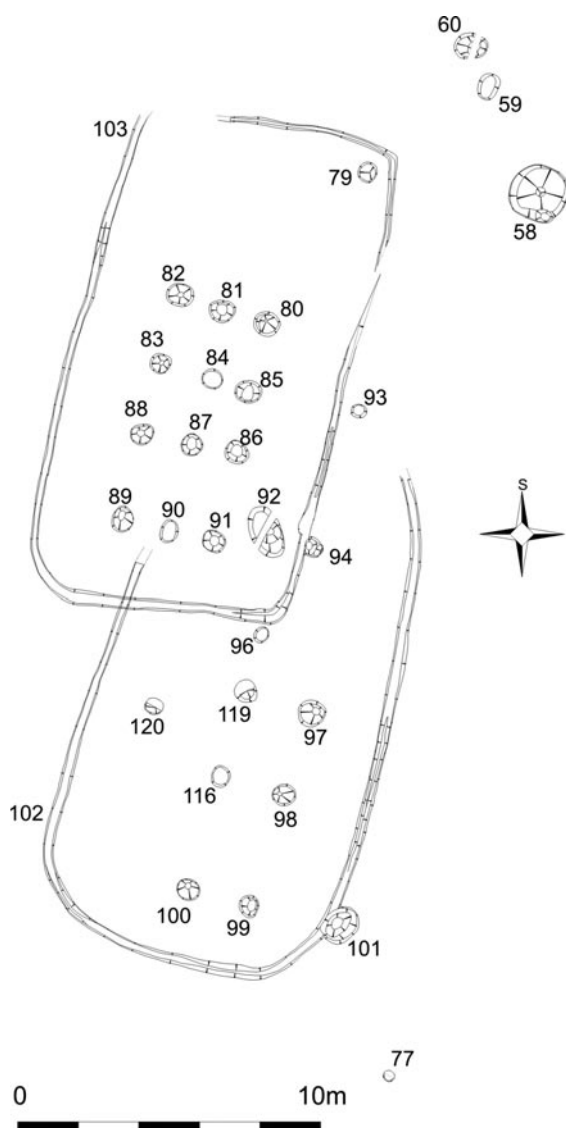
Obr. 7. Čestlice, okr. Praha-východ, poloha K Benicím. Půdorys kúlového domu
