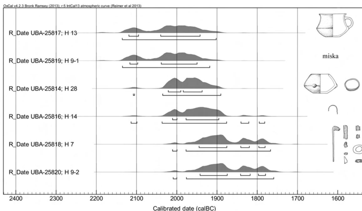
Obr. 22. Přemyslení, okr. Praha-východ. Grafické znázornění výsledků absolutních dat po kalibraci
